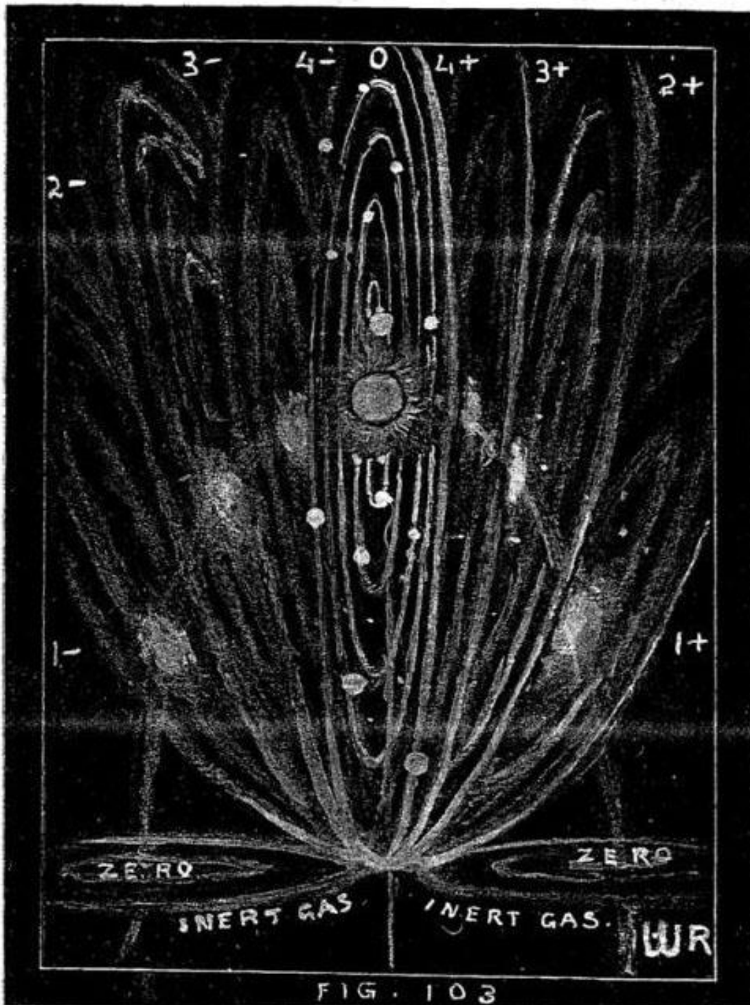
LE SOLEIL CENTRAL DE TOUT SYSTÈME, QUE CE SOIT D'UN ATOME DES ÉLÉMENTS OU D'UN SYSTÈME SOLAIRE DANS NOTRE VOIE LACTÉE, SI À L'AMPLITUDE DE SON ONDE ET À 90 DEGRÉS DE SON AXE D'ONDE, EST UNE VRAIE SPHÈRE ET TOUTES SES PLANÈTES TOURNENT SUR LE PLAN DE L'ÉQUATEUR DE LEUR SOLEIL.
