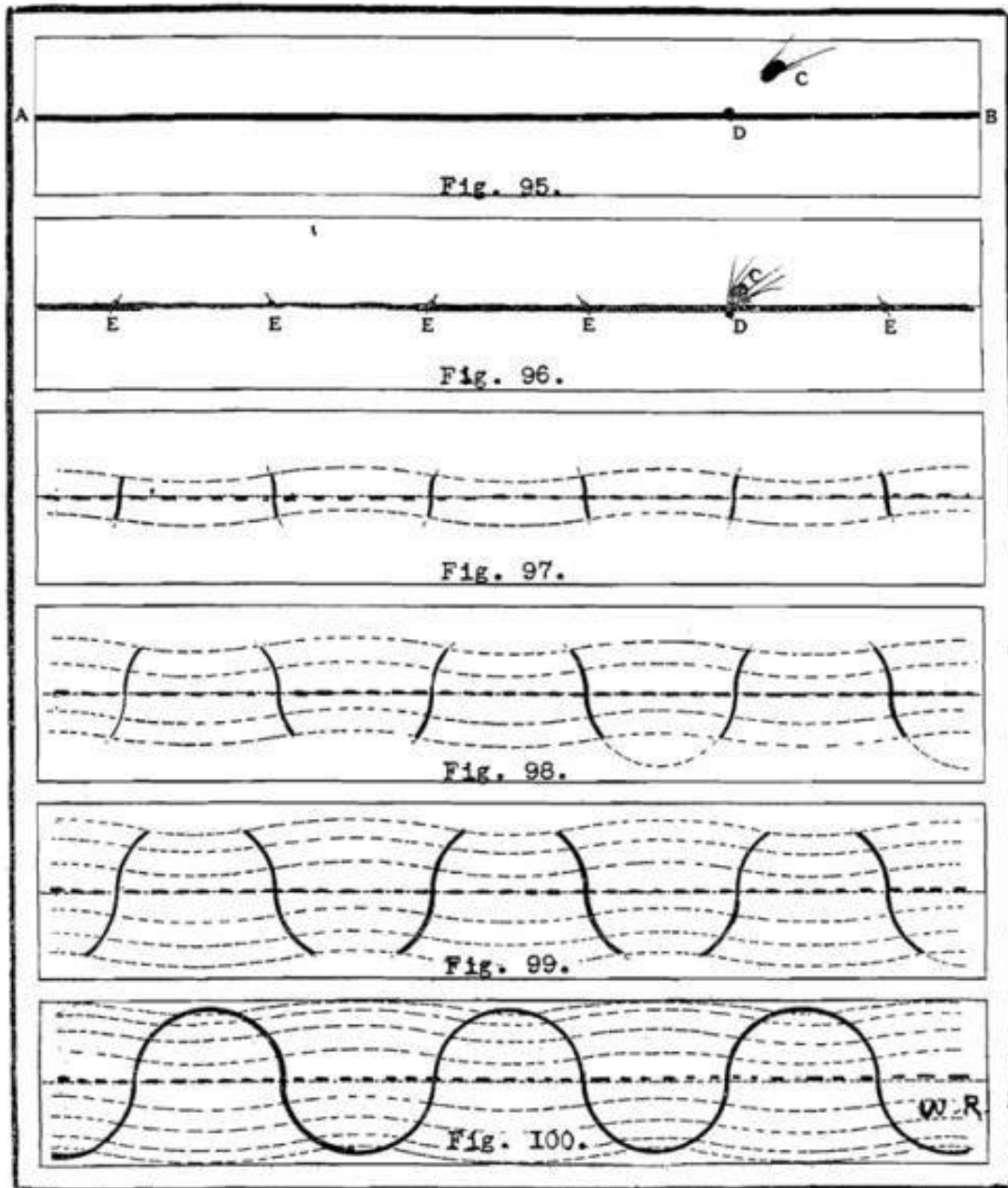
MONTRANT COMMENT L'UNIVERS D'ONDE COURBE DU MOUVEMENT SURGIT DES ÉQUATEURS DE COURBURE NULLE ET RETOURNE À SON IMMOBILITÉ.
