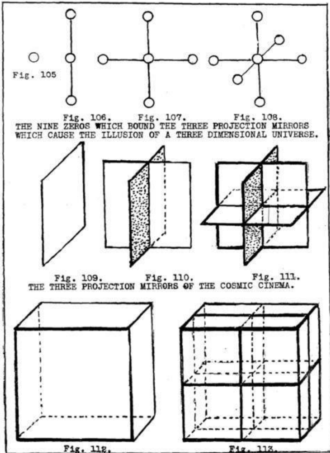
FIG. 112 --- LES SIX MIROIRS DE L'ÉCRAN SPATIAL SUR LEQUEL LE THÉÂTRE COSMIQUE DE LA CRÉATION EST JETÉ.
